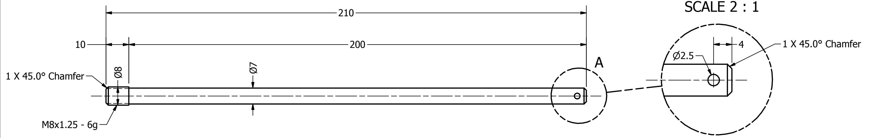
Stang med gevind SCALE 1 : 1
